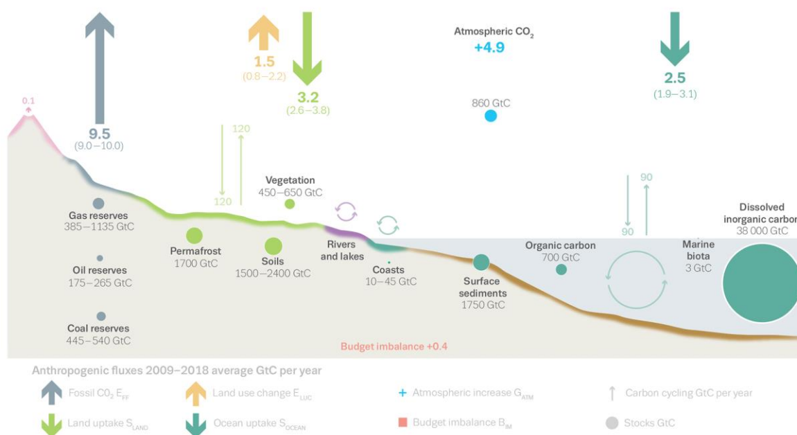
Slika 4: Vpliv človeka na globalno kroženje ogljika (Vir: Pierre Friedlingstein, Matthew W. Jones, Michael O'Sullivan idr.; uporabljen v skladu s CC BY-SA 4.0)
