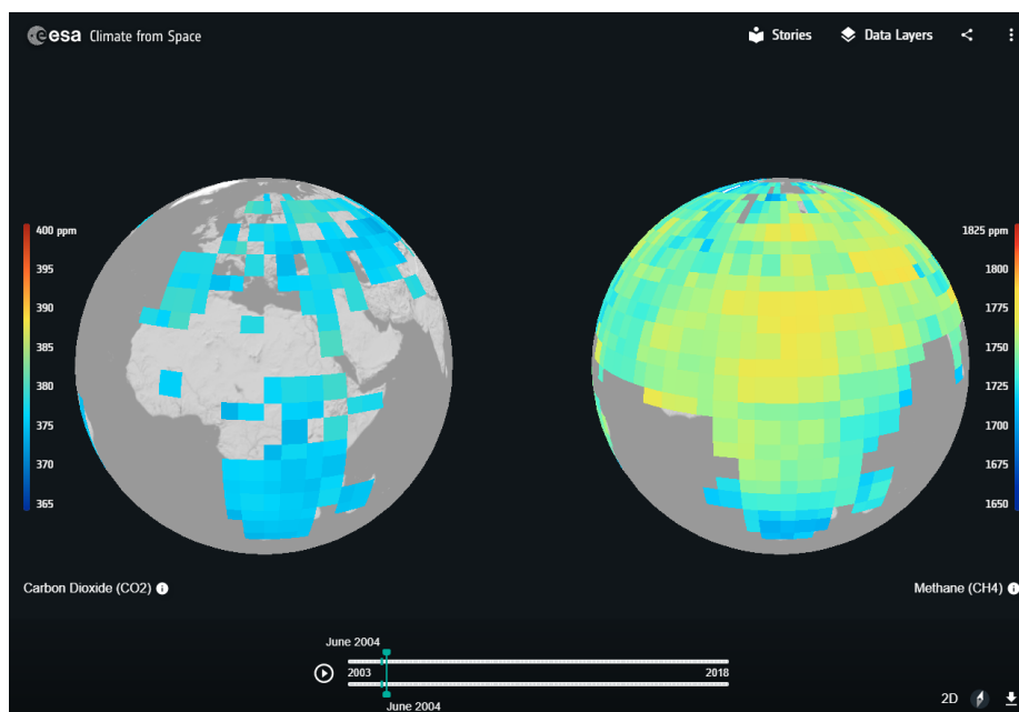
Slika 2: Primerjava podatkov o ogljikovem dioksidu in metanu v spletni aplikaciji Climate from Space (Vir: ESA CCI)
